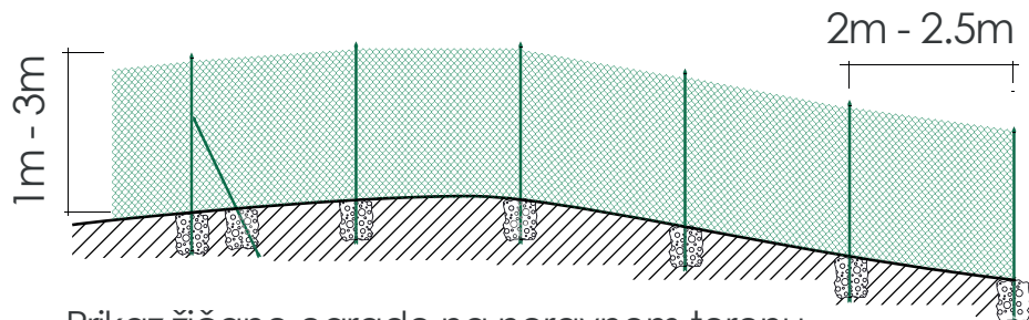
Prikaz žičane ograde na neravnom terenu
